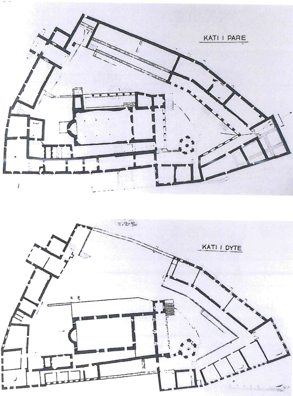
Fig. 5 – Planimetrit e Manastirit
