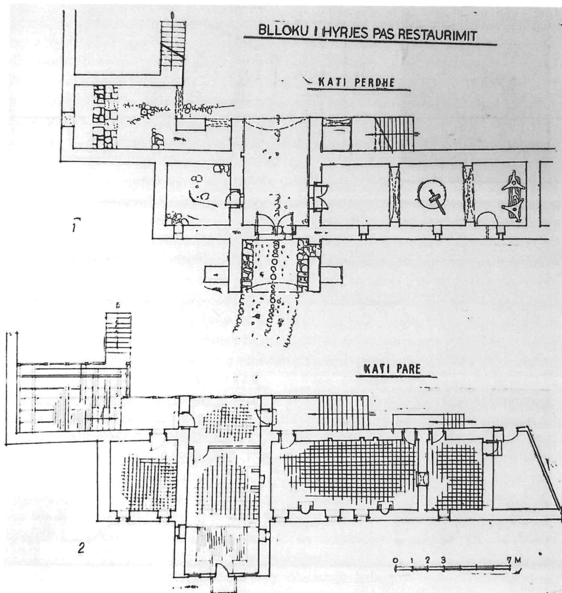
Fig. 7 – Planimetrit e bllokut të hyrjes
