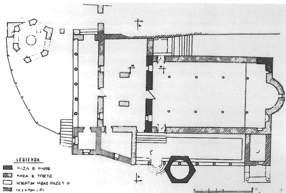
Fig. 8— Planimetri; fazat e ndërtimit kisha e Fjetja e Shën Mërisë
