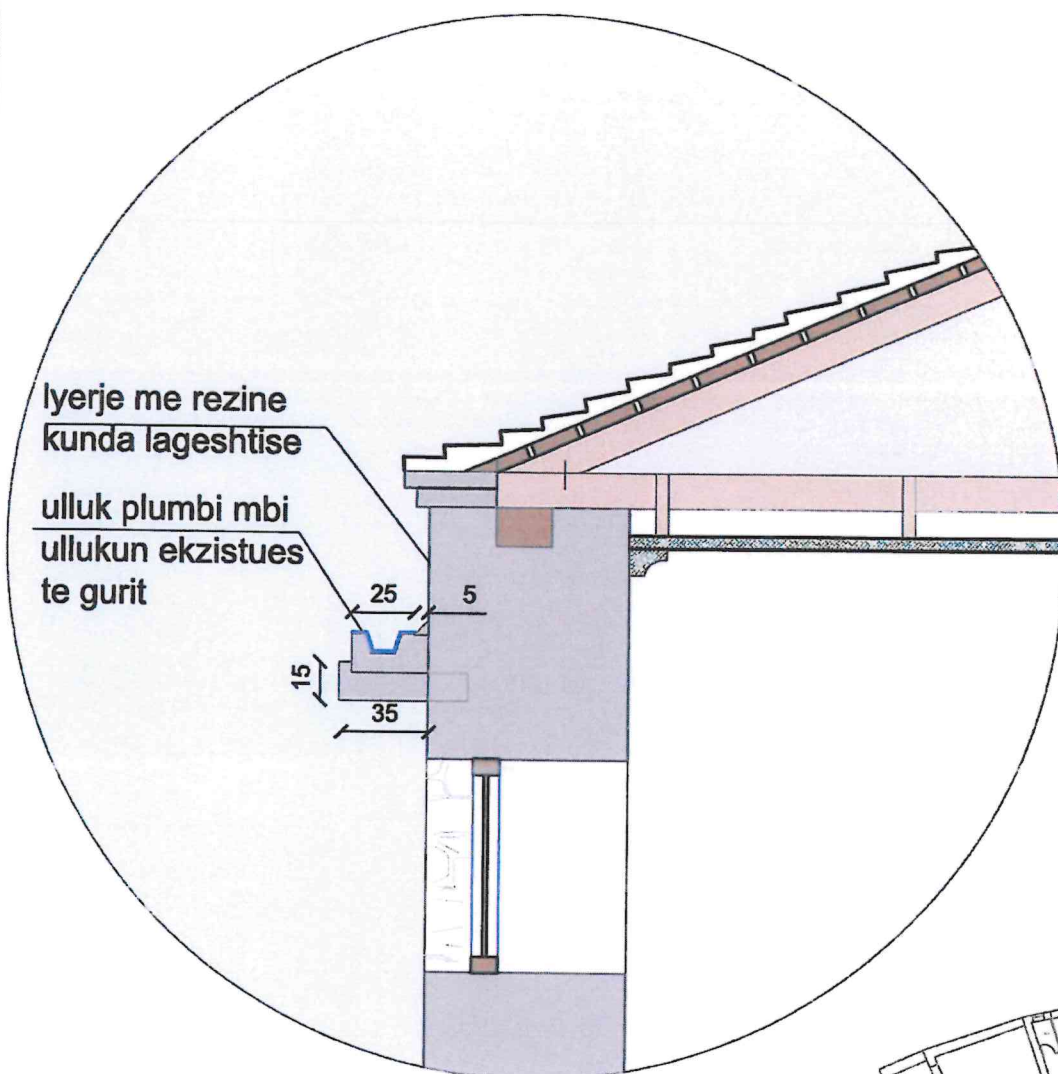
DETAJ I ULLUKUT PREJ PLUMBI MBI ULLUKUN EKZISTUES PREJ GURIT
