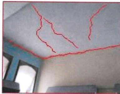
CARËS NË NIVELIN E TAVANIT DHE MURATURES PËR SHKAK TË VËRRIMIT TË FORCESËS SËMË DHE LUNDËS JË TË MËRË MURATURE TAVANË
