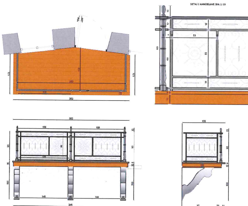
DETAJ BALLKONI Shk.1:25
