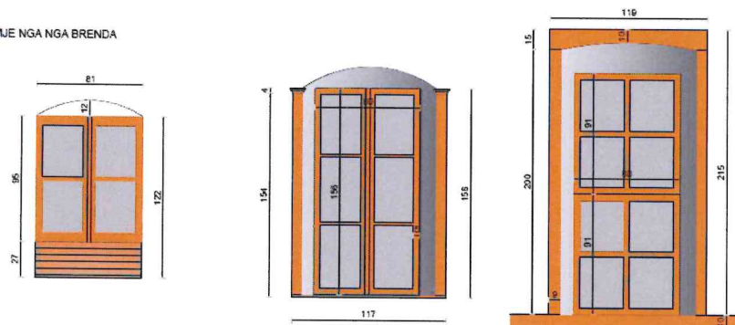
DETAJ BALLKONI Shk.1:25
