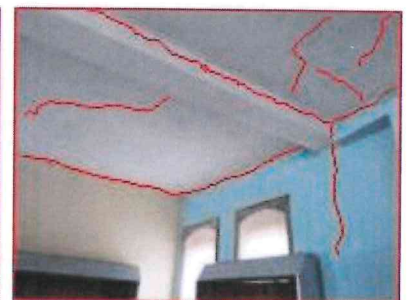
CARËS NË NIVELIN E TAVANIT DHE MURATURES -CARËS NË FUSËN E MURATURES PËR SHKAK TË NËRVOHËMIT TË LUNDË TË MURATURES -CARËS NË FUSËN E SUVASË
