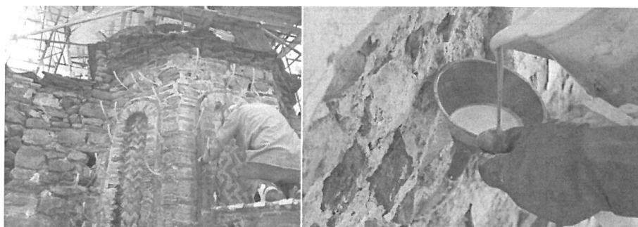
Foto 10. Shembull i procesit të konsolidimit të muraturës
