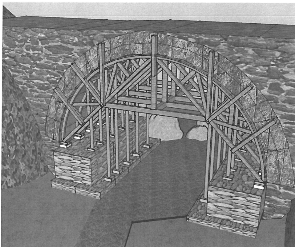
Fig.5- Pajantimi i urës
