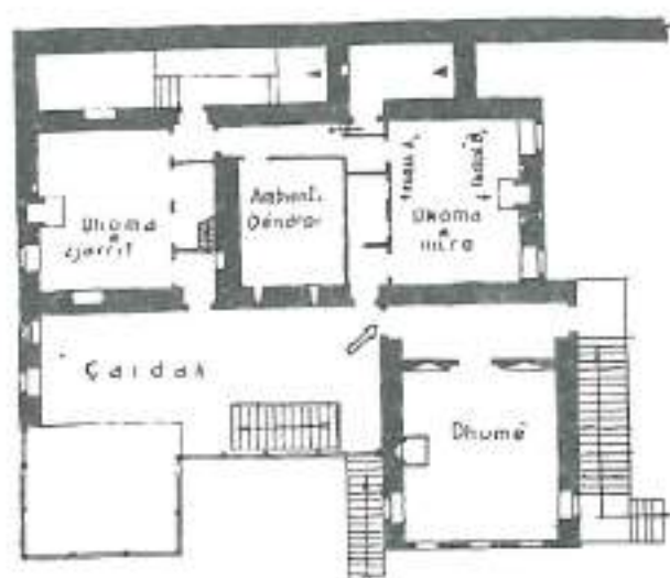
PLANIMETRIA E KATIT I
