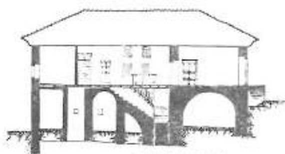
FAȚA LATERALĂ
