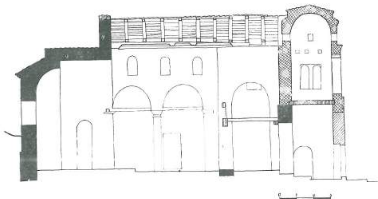
Prerje Gjatësore
