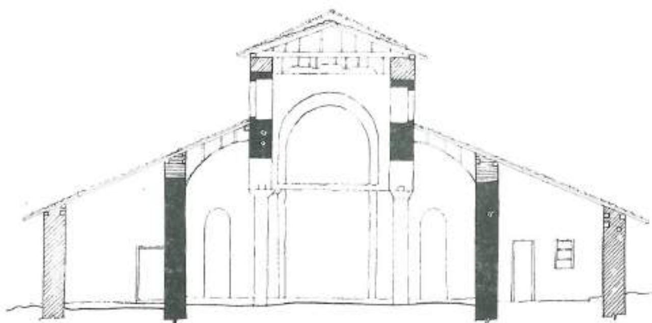
Prerje Terthore
