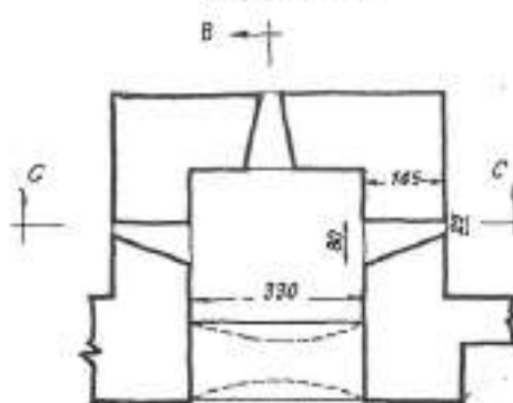
KULLA IV
