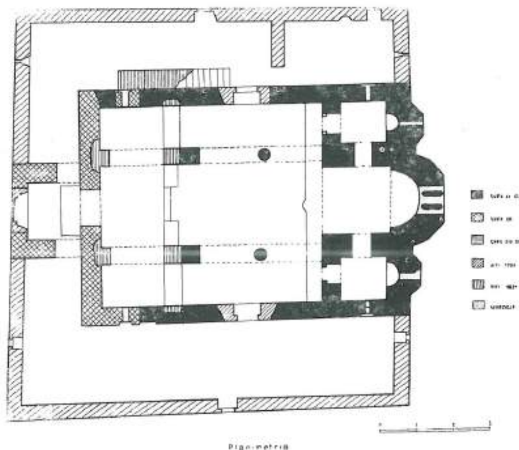
Planimetria
